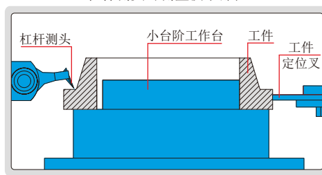
杠杆测头可测量狭小部位
